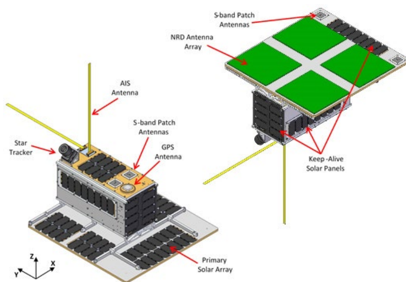
Рис. 2.3. Конструктивная схема ИСЗ NORSAT-3
