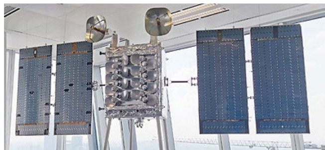
Рис. 2.9. Вид технологического ИСЗ YINHE-1
