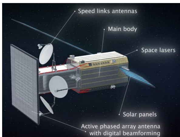
Рис. 2.7. Возможное конструктивное исполнение ИСЗ системы Yaliny
