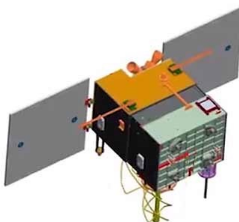
Рис. 2.9. Конструктивная схема ИСЗ TIANQI-8
